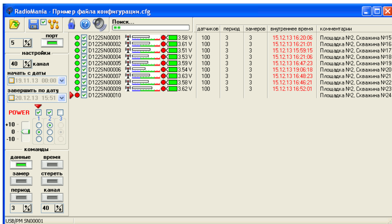
Рисунок 14 – ПО «RadioMania»
