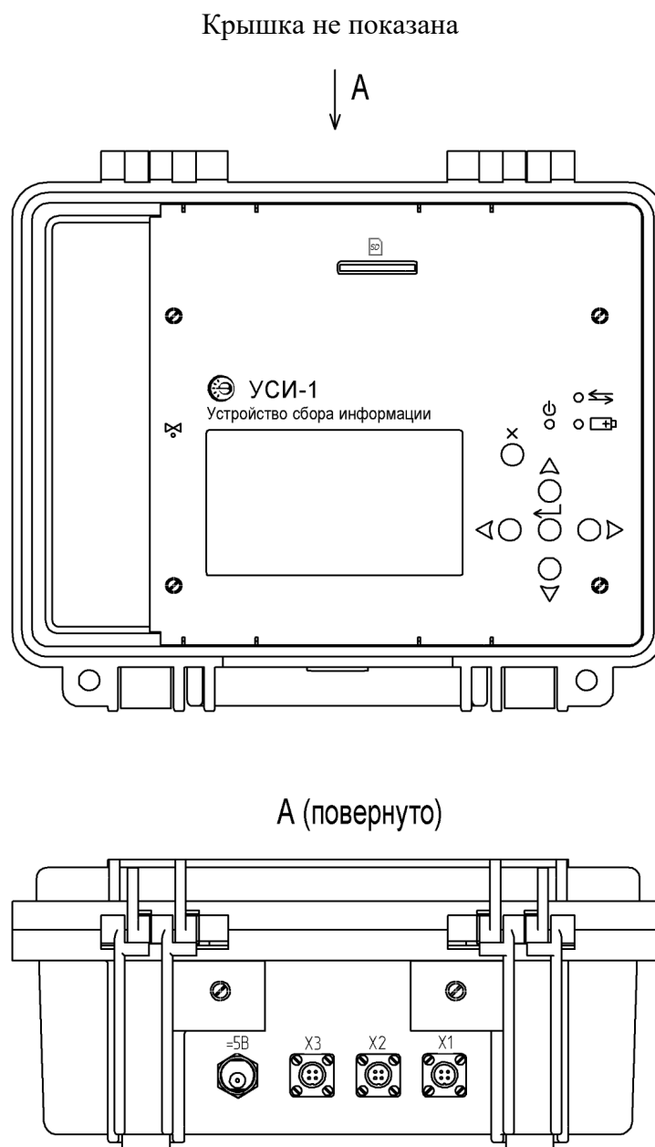
Рисунок 1 – Внешний вид УСИ-1
