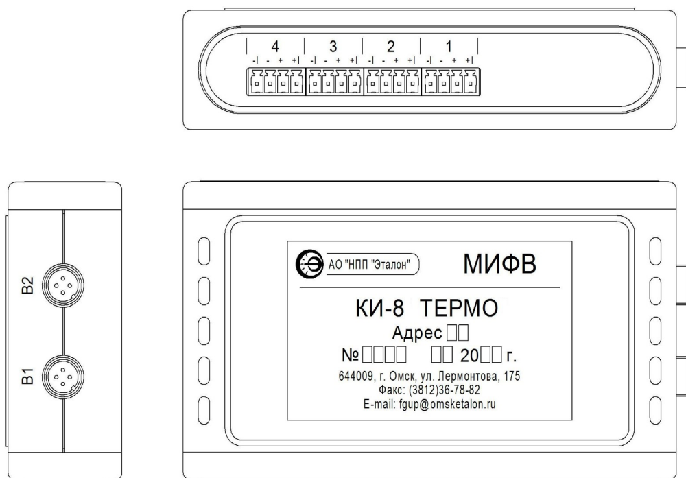
Рисунок 2 – Внешний вид коммутатора измерительного КИ-8 ТЕРМО
