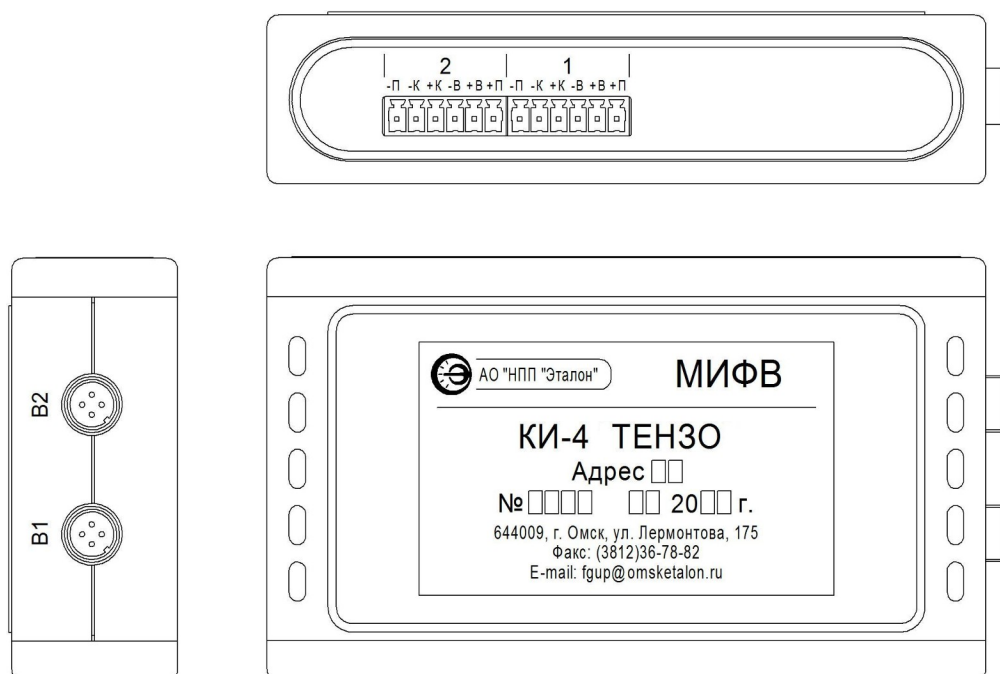
Рисунок 3 – Внешний вид коммутатора измерительного КИ-4 ТЕНЗО
