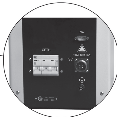
Печь ПРТ 600-1100-2
