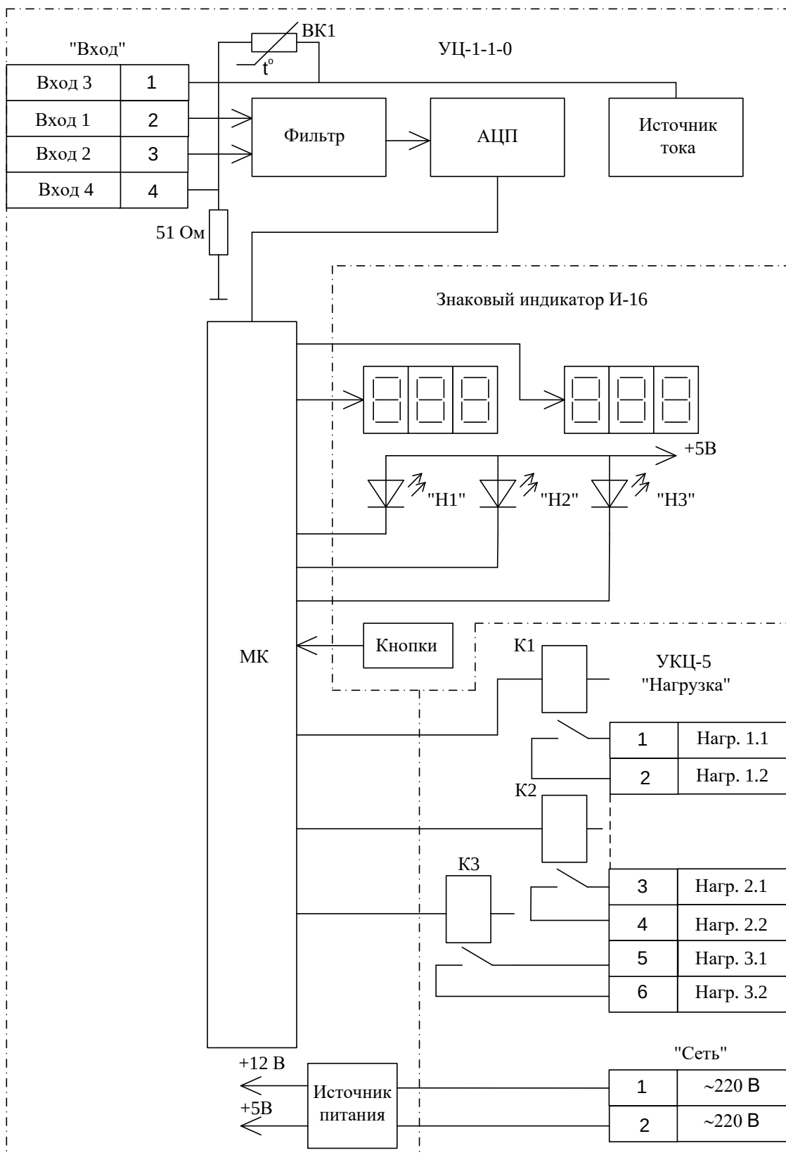
Рисунок 2 – Функциональная схема регулятора
