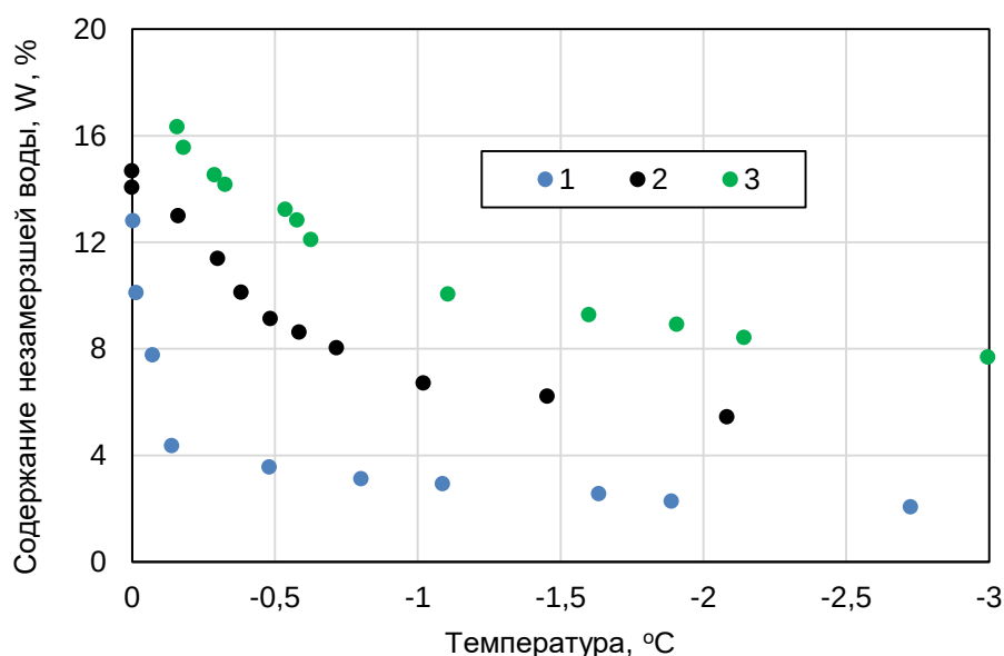
Рис. 1. Изменение содержания незамерзшей воды в области высоких отрицательных температур (до -3^{\circ}\text{C} ) в супесчано-суглинистых грунтах (г. Салехард) с различным содержанием органического вещества ( I_r ): 1- 0,94%, 2 – 1,76%, 3 – 5,51%.
