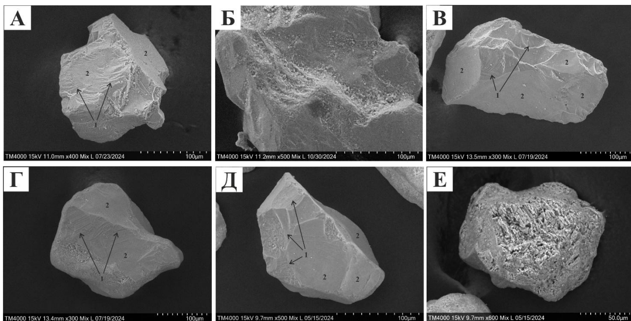
Рис. 1. Криогенный микрорельеф песчаных зёрен кварца: 1 – раковистые сколы, 2 – гладкие полированные поверхности (А – песчаное зерно из водноосадочных отложений; Б – увеличенный фрагмент раковистых сколов (водноосадочные отложения); В, Г, Д, Е – песчаные зёрна из субаэральные отложений).
