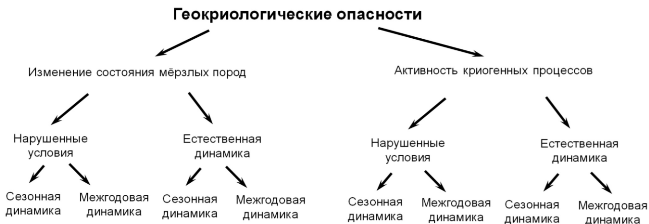
Рис. 1. Структура понятия геокриологической опасности.
